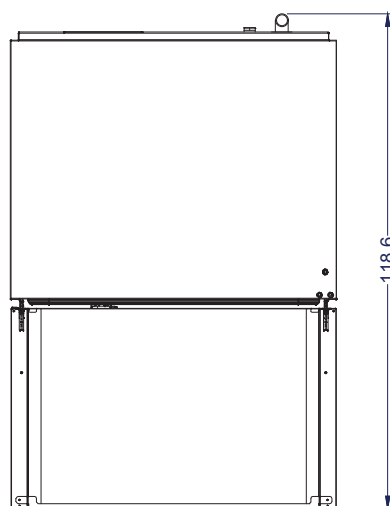
Vista Planta
