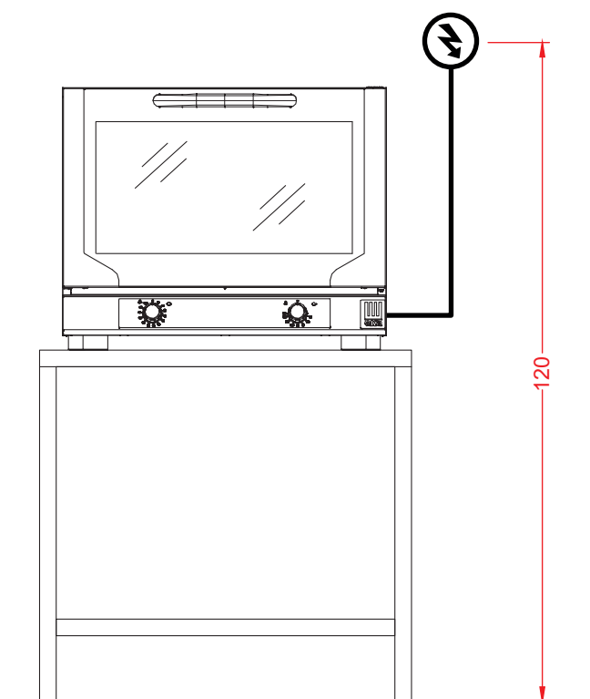
Vista Elevación
